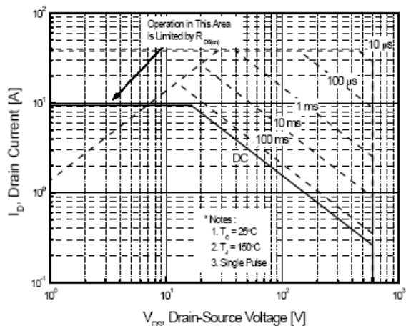
图 6-3 10N65(TO-262&263)
