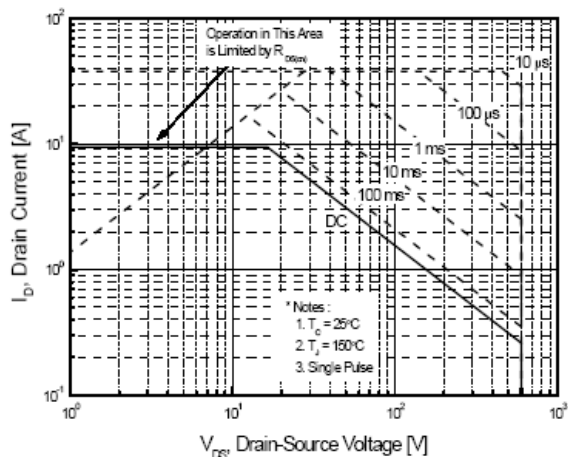
图 6-1 10N65(TO-220)
