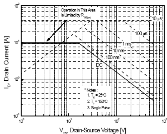
图 6-1 10N65(TO-220F)
